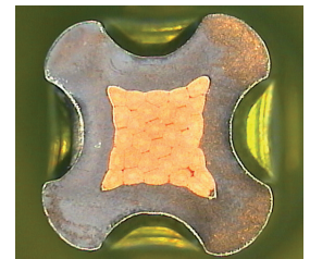
Querschnitt eines Vierdorncrimps Cross-section of a four-indent crimp
